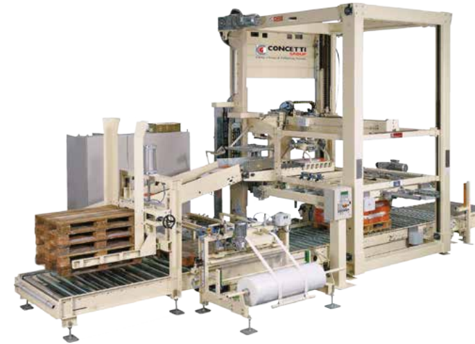
Palettiseur robotisé :
