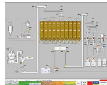
Page du panneau opérateur, Gestion de l'installation complète
