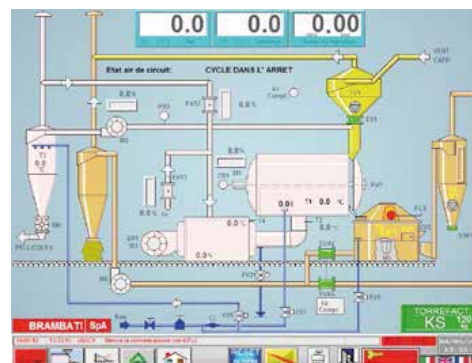
Page du panneau opérateur, Gestion du torréfacteur
